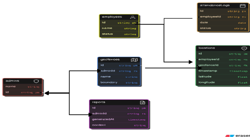
ER Diagram
